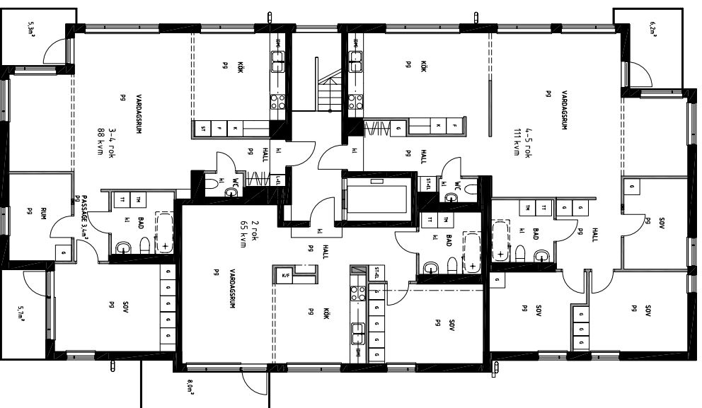
HUS 4 NORMALPLAN 1:200
